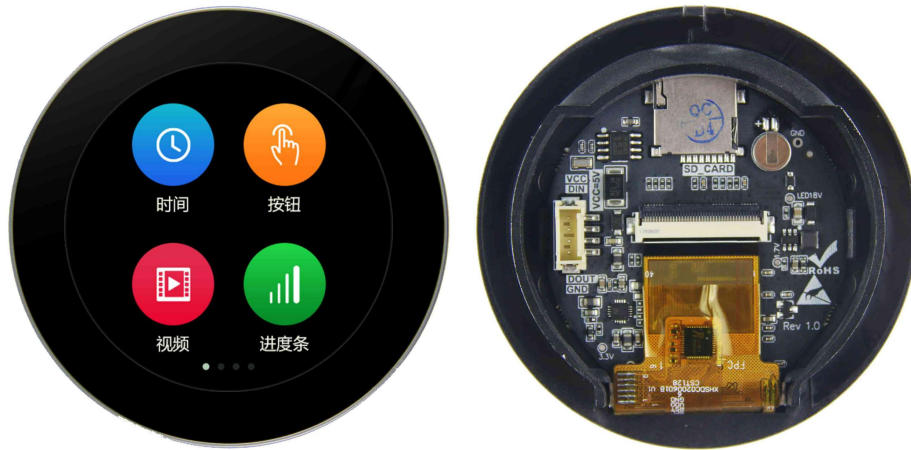
图 1-1 2.1 寸电容触摸参考图
