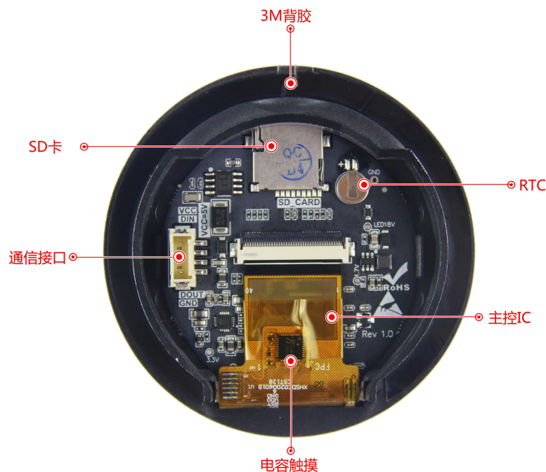
图 1-2 硬件配置图
