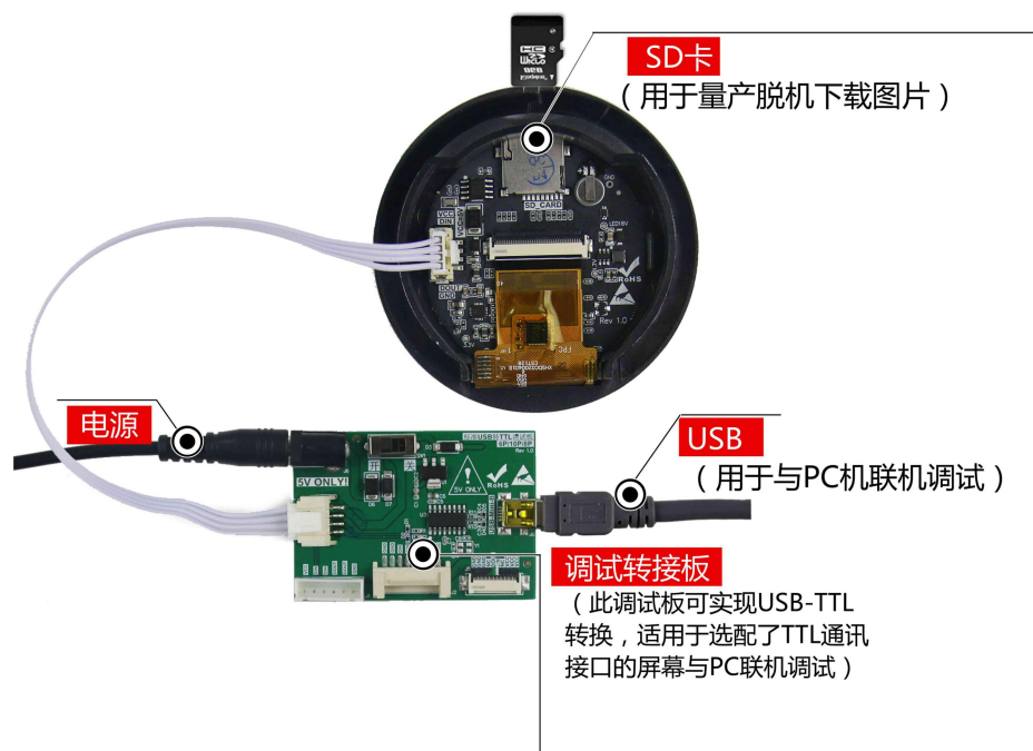
图 1-3 TTL 调试工具图
