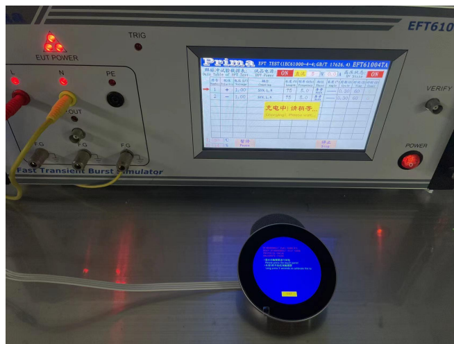
图 6-4 群脉冲测试图
